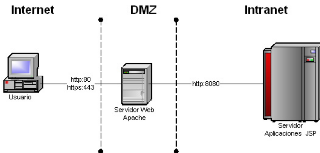
1. Esquema básico de arquitectura Web.
